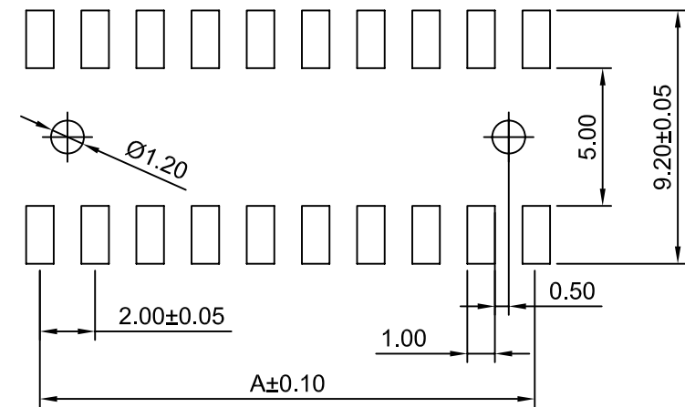
P.C.B LAYOUT
